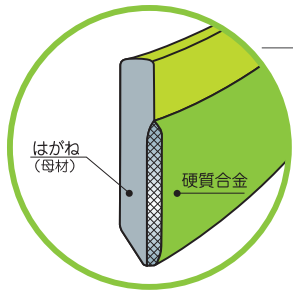
快適Z爪断面図
